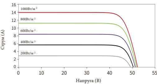
Криві струм-напруга (72HL4-BDV 580Вт)
