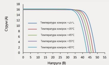
Струм-напруга (615 Вт)
