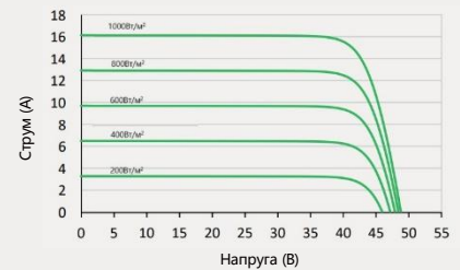
Потужність-напруга (615 Вт)
