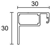
Переріз рами В-В
